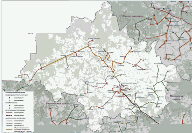
Схема газоснабжения и газификации Мосальского района Калужской области
