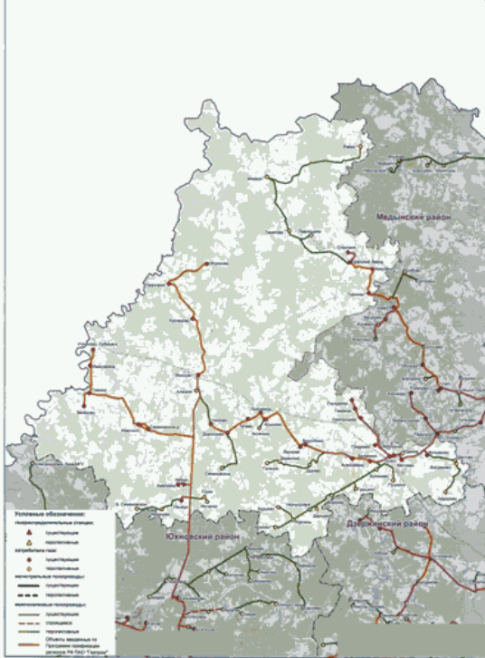
Схема газоснабжения и газификации Истринского района Калужской области
