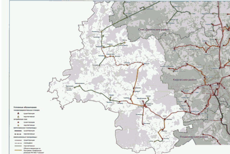
Схема газоснабжения и газификации Куйбышевского района Калужской области
