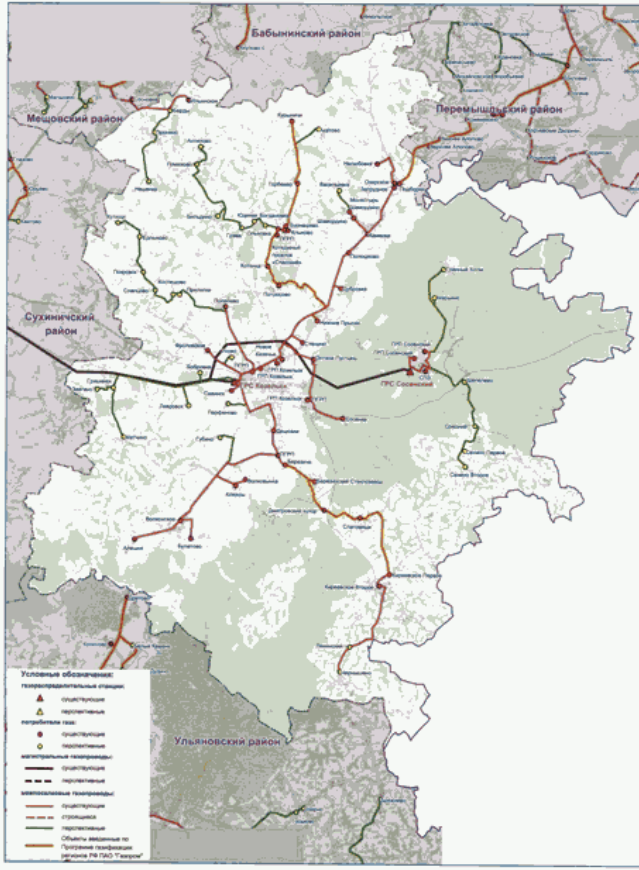
Схема газоснабжения и газификации Козельского района Калужской области
