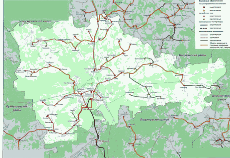
Схема газоснабжения и газификации муниципального района "город Киров и Кировский район" Калужской области
