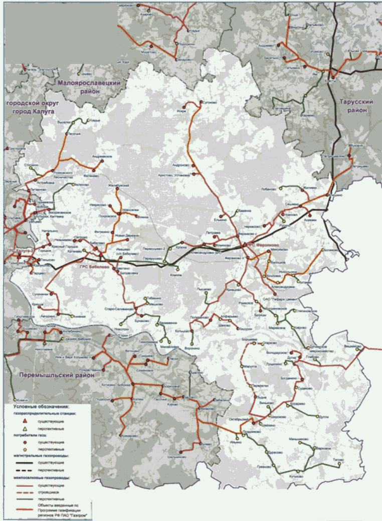
Схема газоснабжения и газификации Ферзиковского района Калужской области
