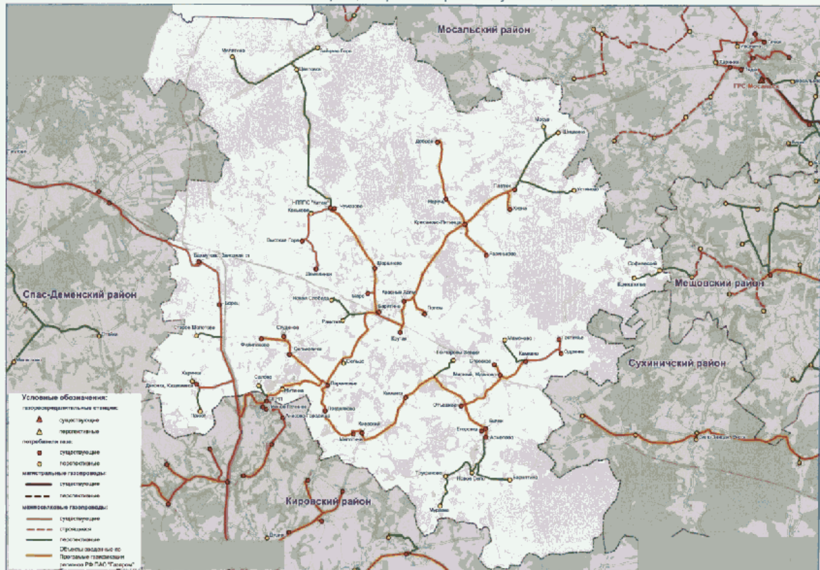
Схема газоснабжения и газификации Барятинского района Калужской области
