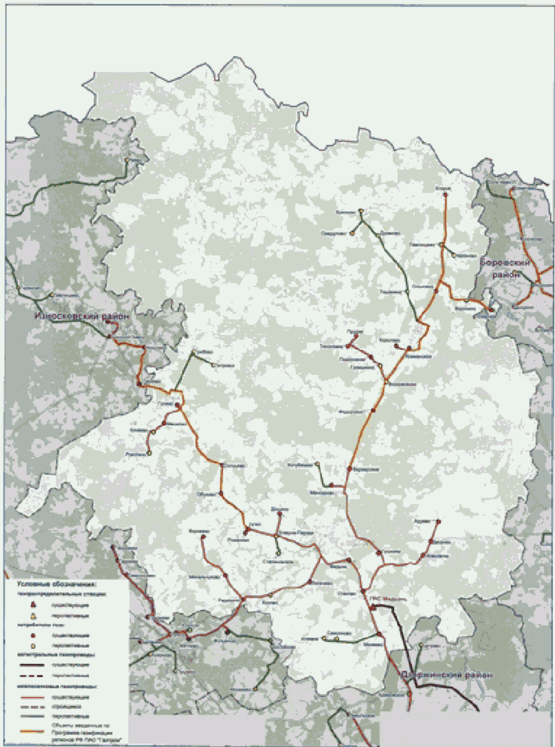
Схема газоснабжения и газификации Медынского района Калужской области
