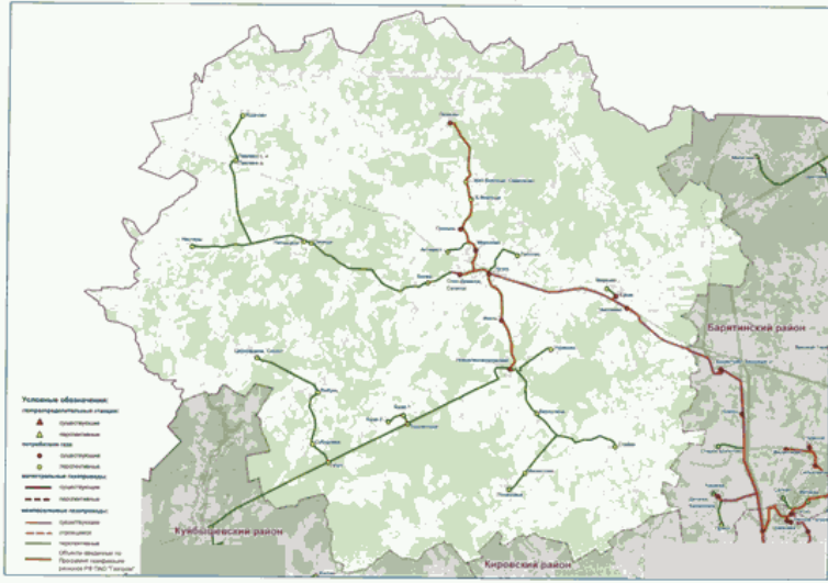
Схема газоснабжения и газификации Спас-Деменского района Калужской области
