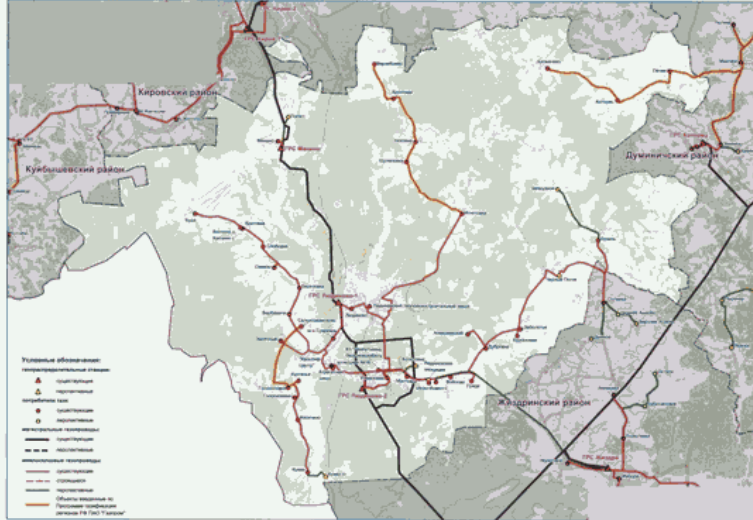
Схема газоснабжения и газификации муниципального района "город Лединово и Лединовский район" Калужской области
