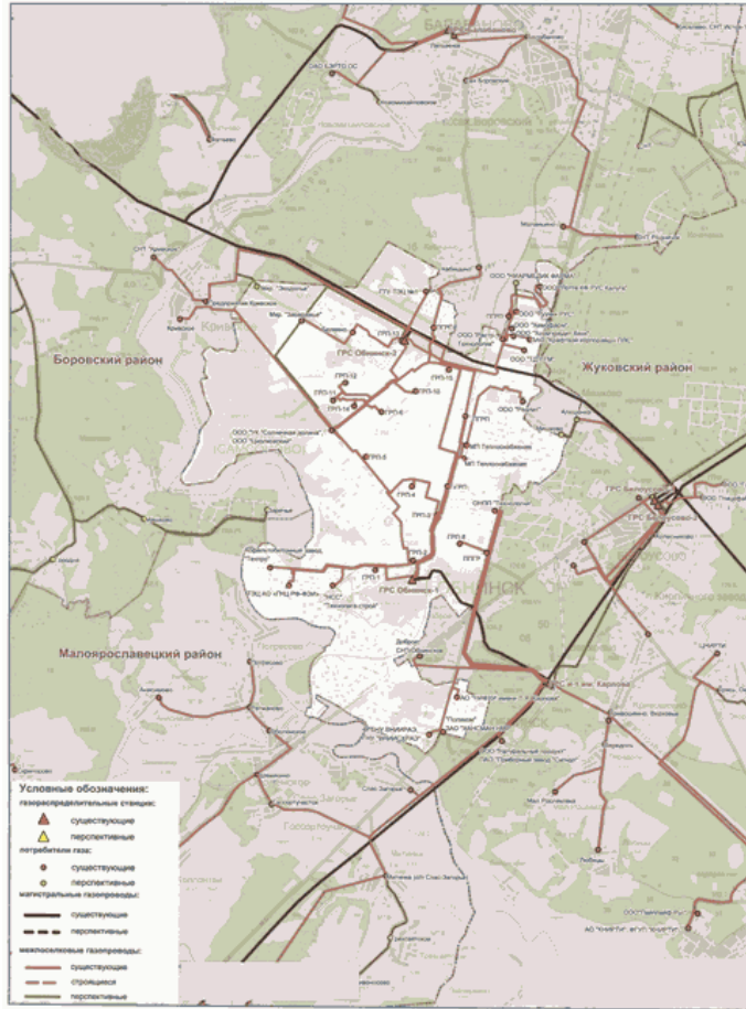
Схема газоснабжения и газификации городского округа "город Обнинск" Калужской области
