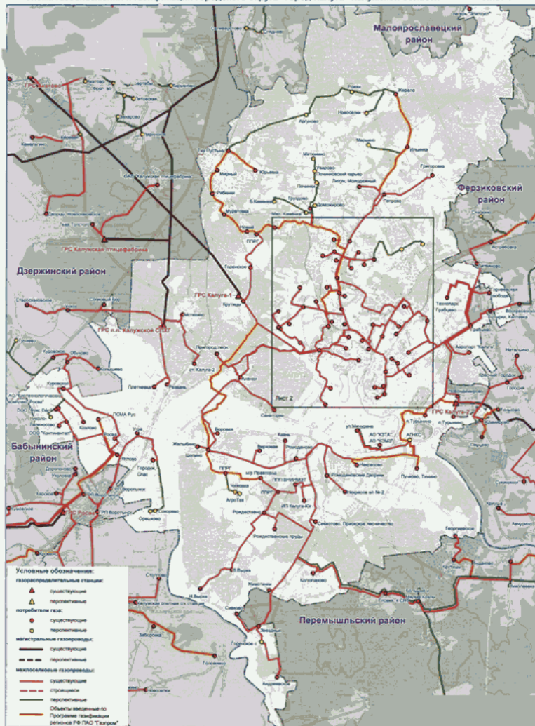
Схема газоснабжения и газификации городского округа "город Калуга" Калужской области - Лист 1
