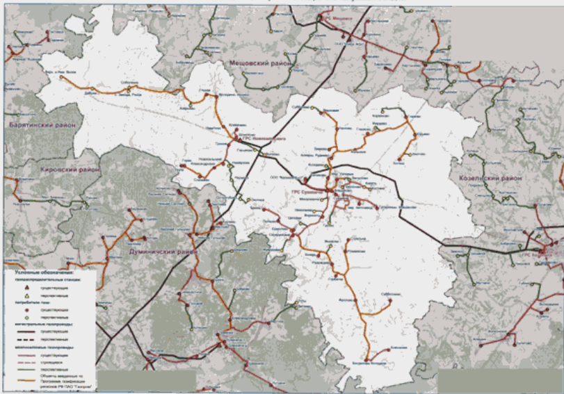
Схема газоснабжения и газификации Сушинского района Калужской области
