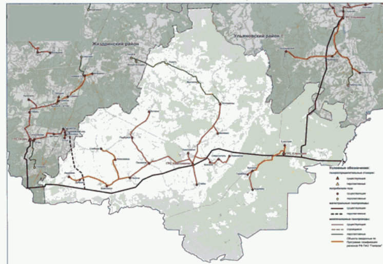
Схема газоснабжения и газификации Хвостовского района Калужской области
