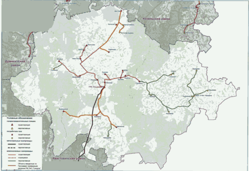
Схема газоснабжения и газификации Ульяновского района Калужской области
