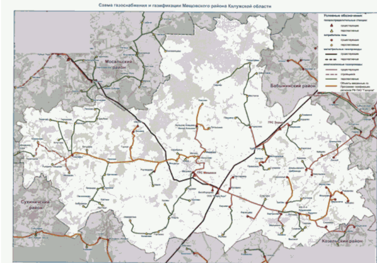
Схема газоснабжения и газификации Мещовского района Калужской области
