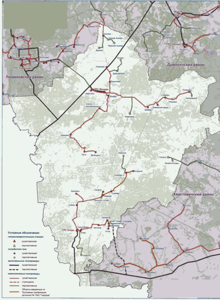
Схема газоснабжения и газификации Жиздринского района Калужской области
