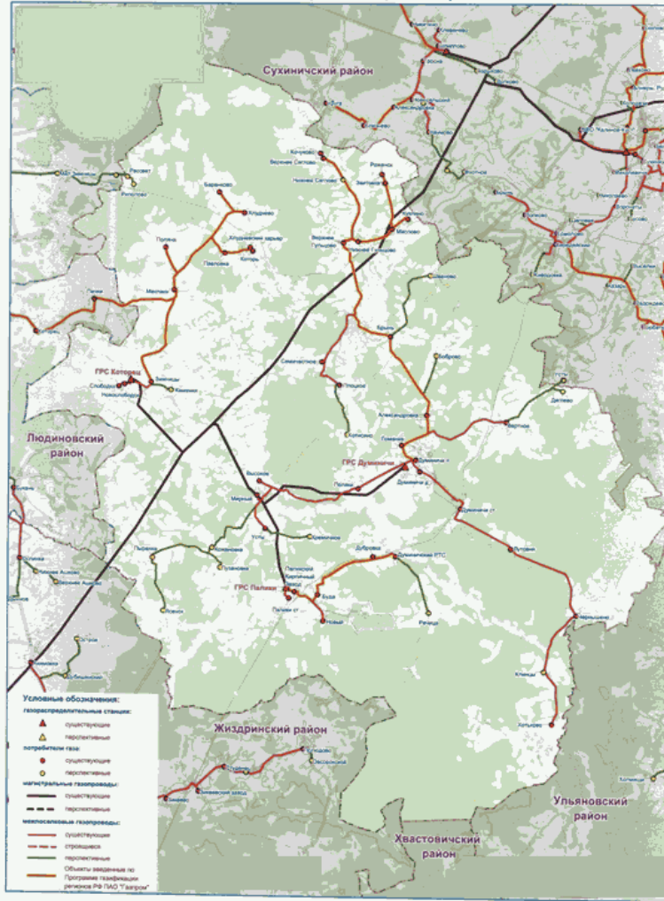
Схема газоснабжения и газификации Думиничского района Калужской области
